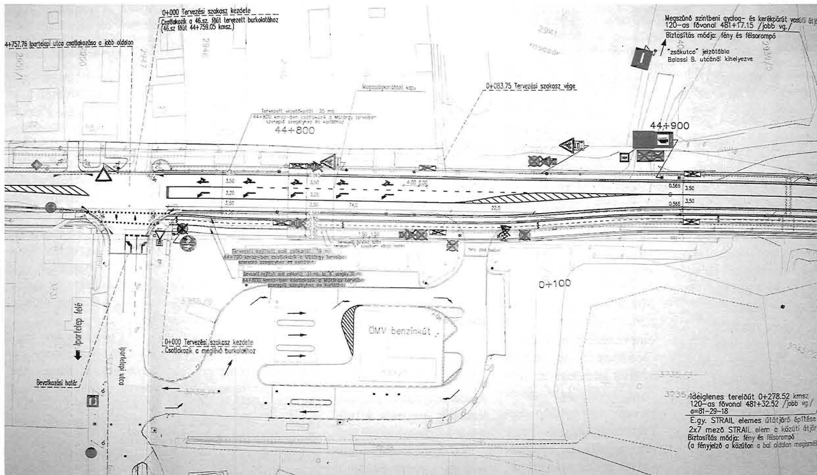
Ipartelepi út csomópontjának (OMV kút) forgalomszervezési terve
