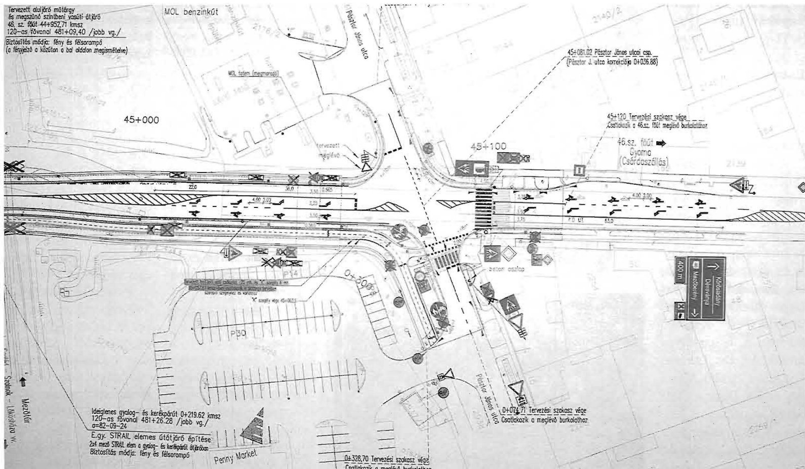
A Fő út - Pásztor János út csomópontjának (MOL kút - Penny Market) forgalomszervezési terve
