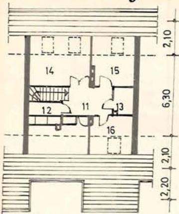
TETŐTÉR ALAPRAJZA M = 1 : 200
