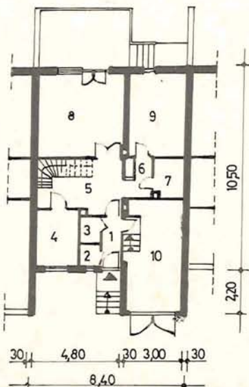
FÖLDSZINT ALAPRAJZA M = 1 : 200
