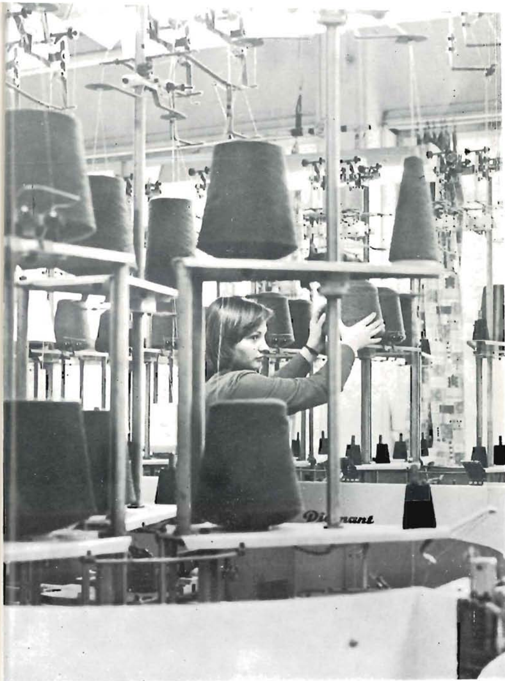
NDK gyártmányú körsikkötőgép
