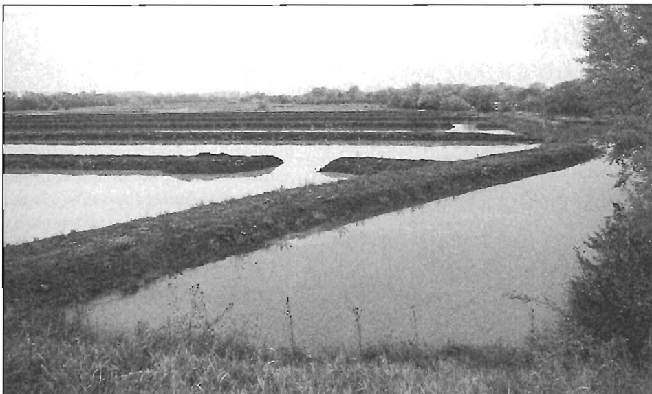
A kiszivattyúzott iszapos víz az ülepítő kazettákon keresztül folyik át
