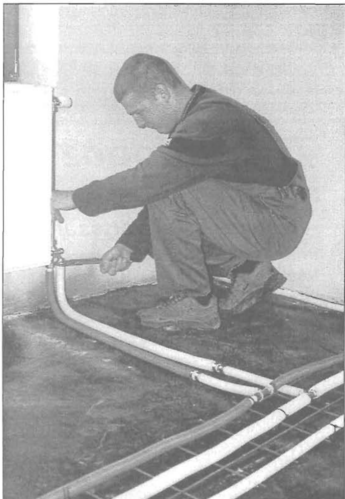
Központifűtés szerelés (Sebők Zsolt - Budai Nagy A. utca)
